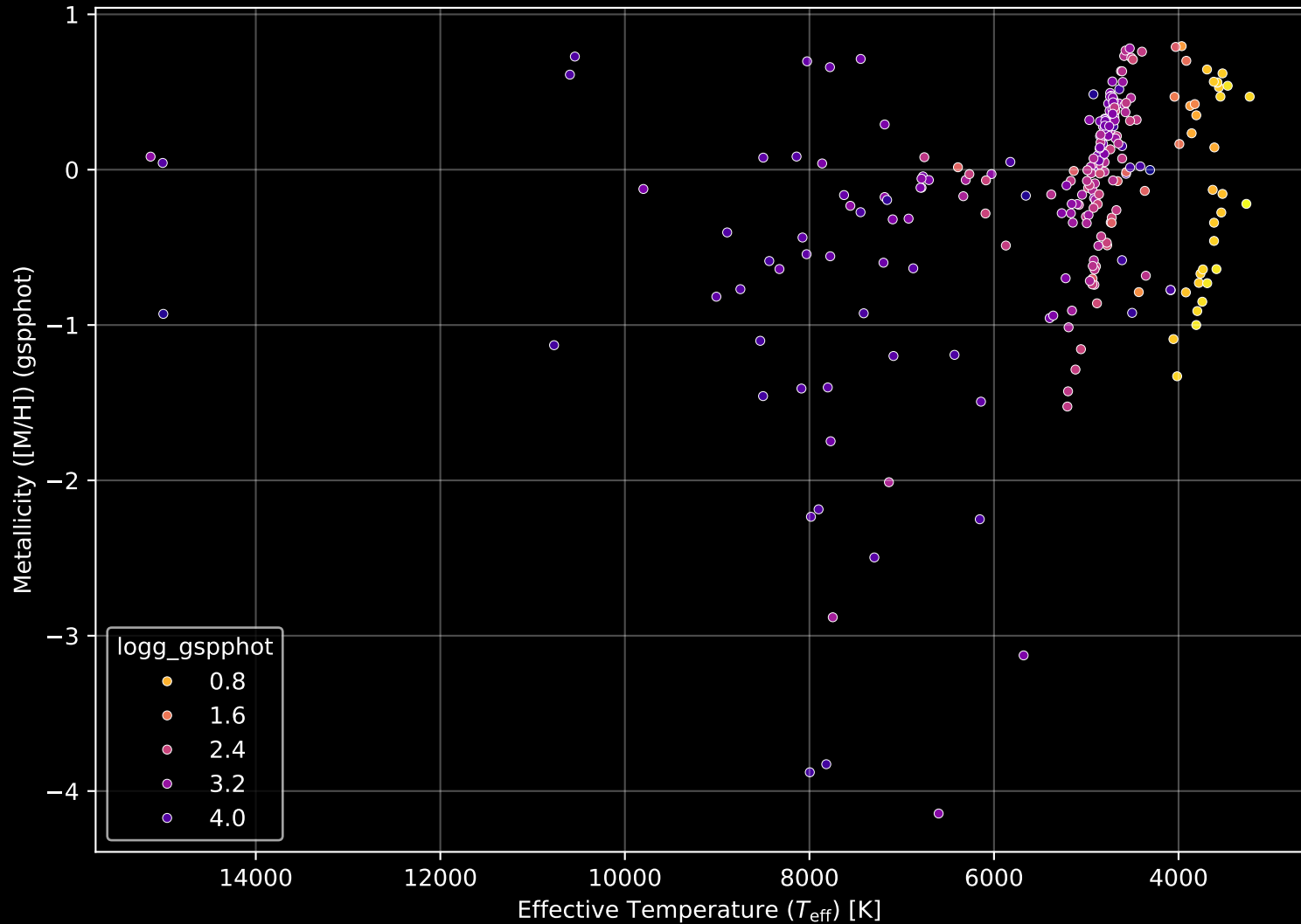
APOGEE DR17 Field: [000+04] Stellar Population Parameters (n= 260)
